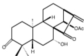
蓝萼乙素
